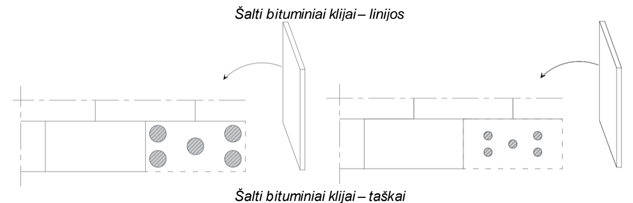
9 9: Montavimas klijuojant – klijavimo būdas (pagrindiniai brėžiniai) 4
