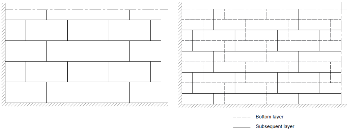
3 3: Klijimas persidengimo būdu (kairėje: vienas sluoksnis; dešinėje: daugiasluoksnis)
